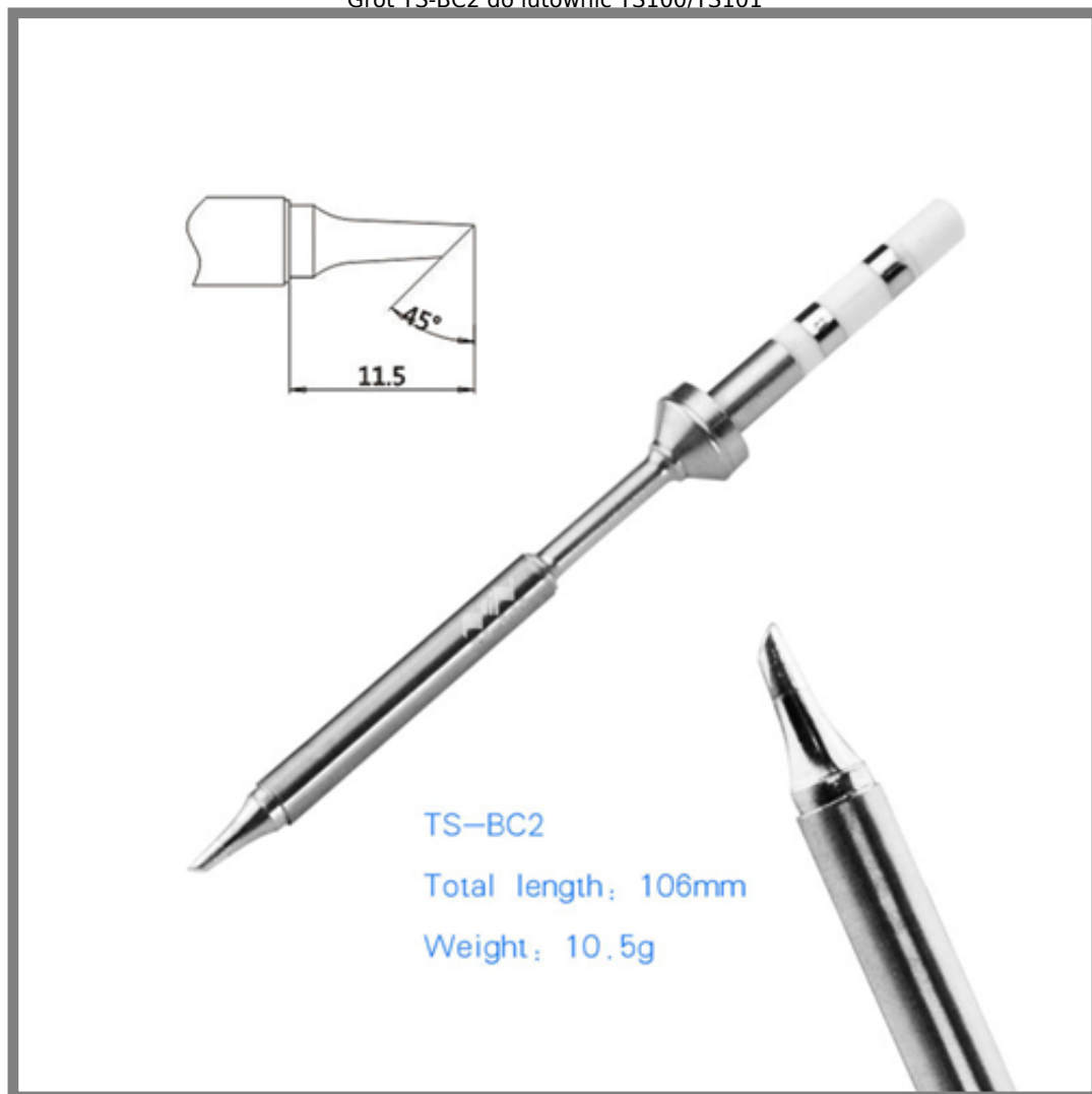
Grot TS-BC2 do lutownic TS100/TS101
